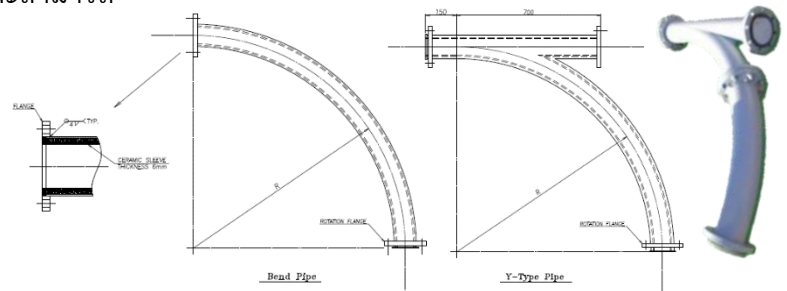
ท่อข้อต่อโค้งเซรามิกไลน์เนอร์
